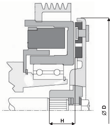
DÍLY SPOJKY - PŘÍTLAČNÝ TALÍŘ S DRÁŽKOVANOU HŘÍDELÍ
