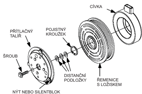
DÍLY SPOJKY - PŘÍTLAČNÝ TALÍŘ S DRÁŽKOVANOU HŘÍDELÍ
