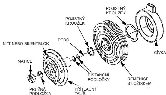
DÍLY SPOJKY - PŘÍTLAČNÝ TALÍŘ S DRÁŽKOU A PEREM
